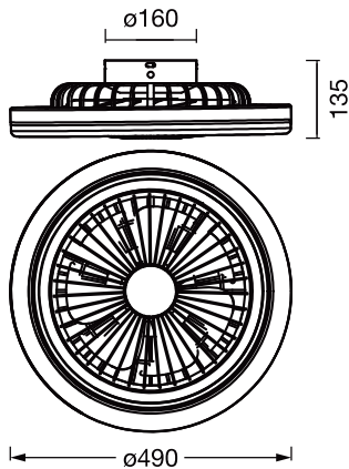
CEILING FAN SOLANO 490 41W CCT
